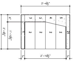
SECTION A-A SCALE: 3/4" = 1'-0"
