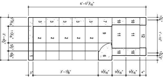
SECTION A-A SCALE: 1" = 1'-0"
